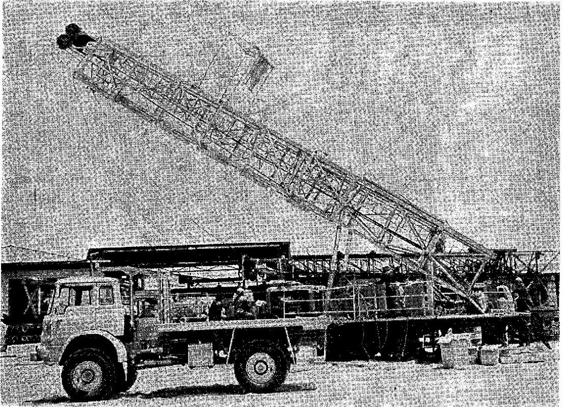
احدى آلات الشركة الحديثة ( ميهيو ٢٠٠٠ ) التي تستطيع ان تصل الى عمق ١٦٠٠ متر
