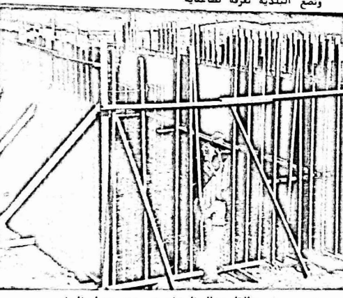
صورة القاعدة الخفية (٤٥٥مx١١مx٣م ارتفاع) وعليها ستترك بواسطة الرميكرات لتقليل الاهتزاز قاعدة المونور العليا (٤٥٥مx١١مx٣م)
